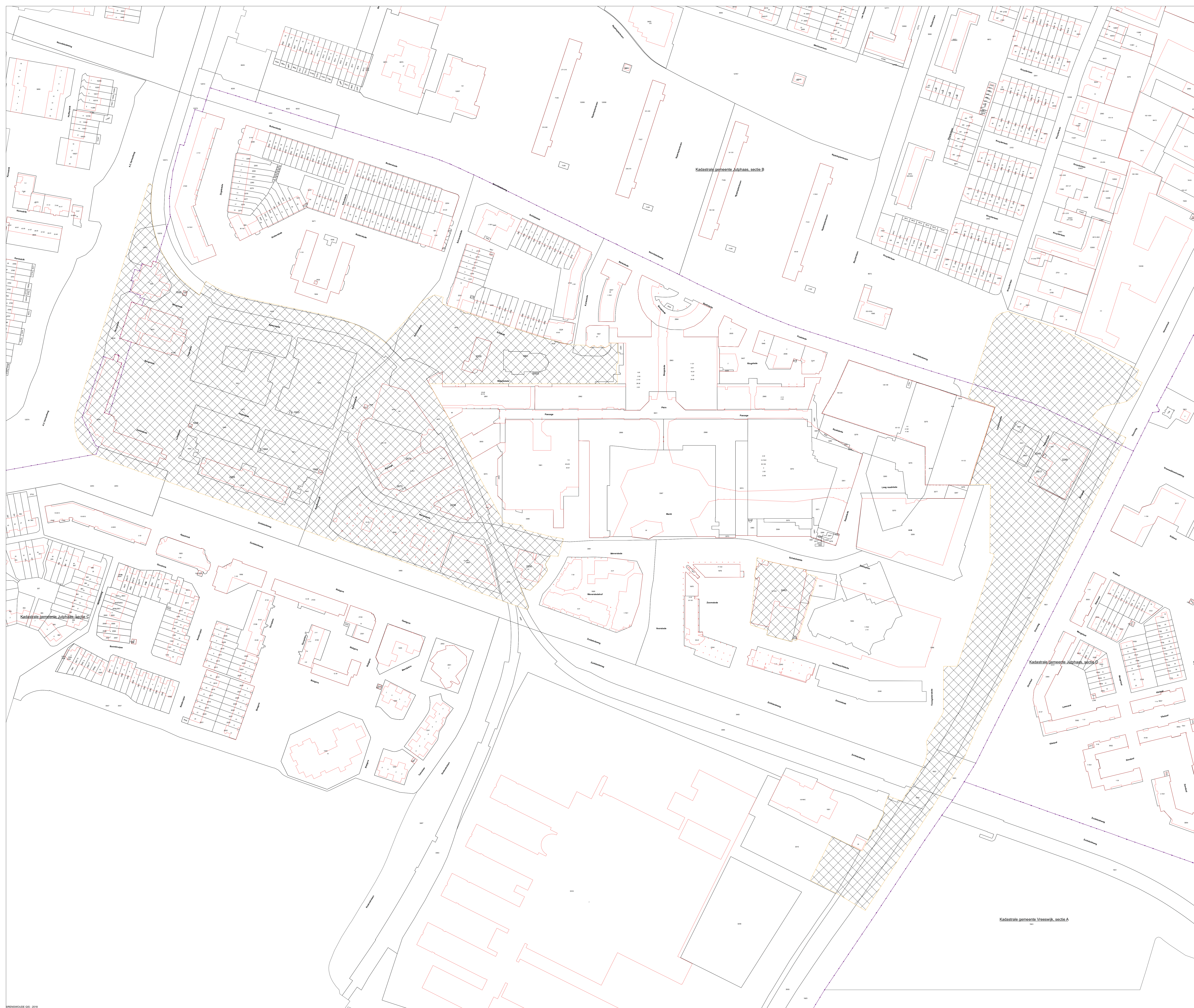
Wvg"City Nieuwegein" te Nieuwegein Masterplantekening
